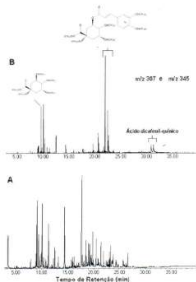
Figura 2: A) Cromatograma de íons totais de um extrato hidroalcoólico de própolis coletada no Estado do Rio de Janeiro. B) Fragmentograma dos íons m/z 307 e m/z 345, característicos do ácido quinico ( t_R 9,6 min) e cafeoil derivados 140 .
