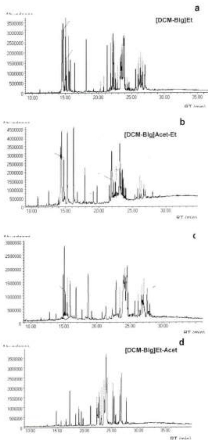
Figura 1. CGAR de frações de própolis avaliadas contra Trypanosoma cruzi 127 .
